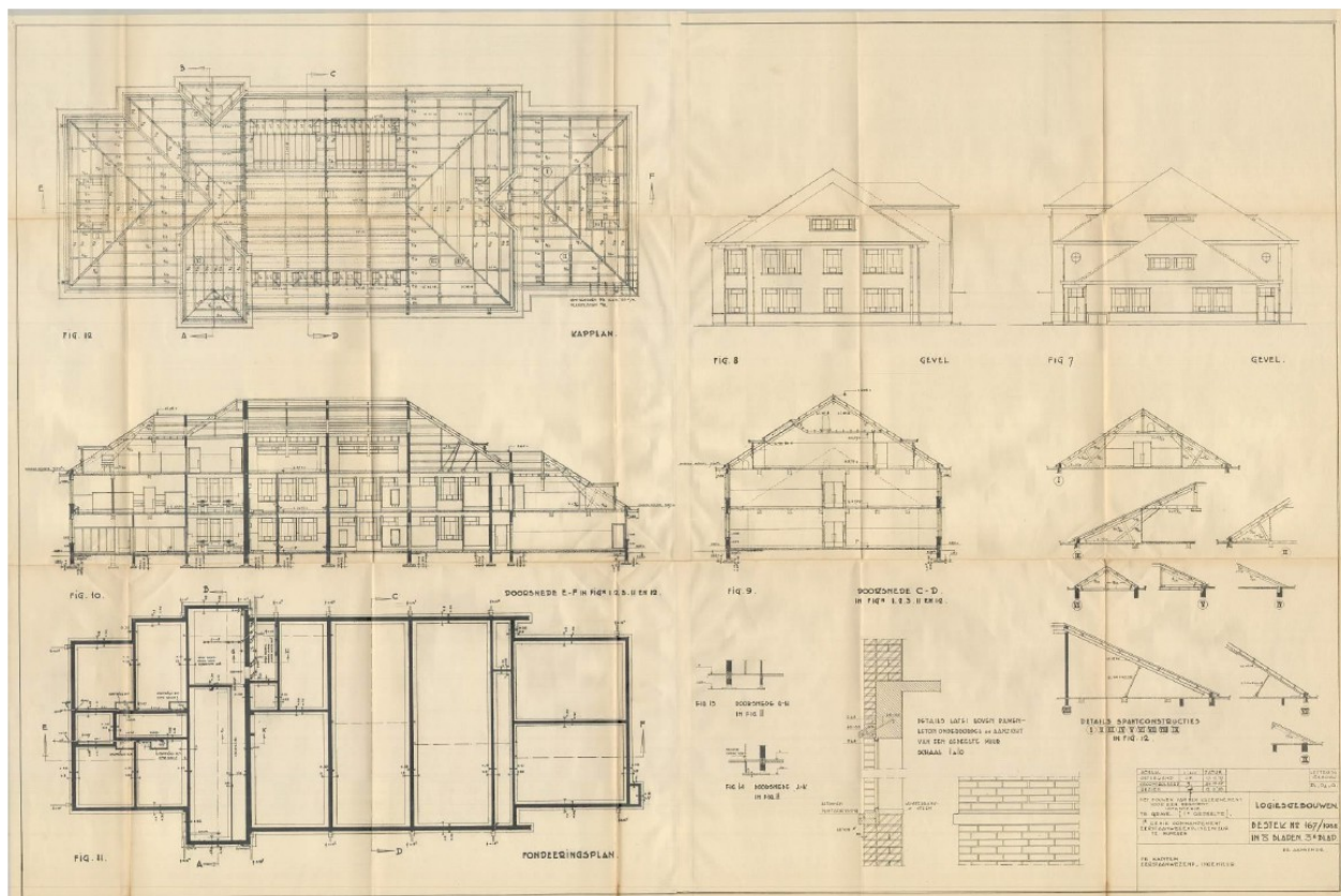
Plattegronden fundering en dakconstructie, doorsneden, kapdetails en kopgevels logiesgebouwen D1, D2 en G. 7-3-1938. BHIC Gemeentebestuur Velp 1814-1942, toegang 7037 Bouwvergunningen 628.02
